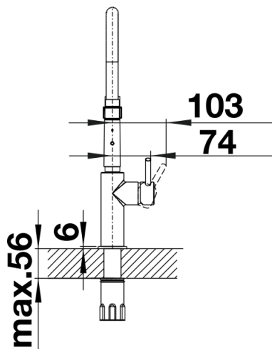
Seitenansicht Hebel 2D
